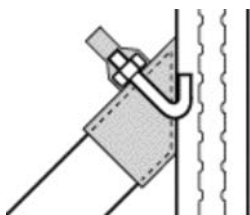
Pfosten mit Strebe
